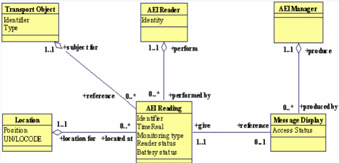
Obrázek 1 – Schéma složek systému AVI/AEI při intermodální/multimodální přepravě nákladu
