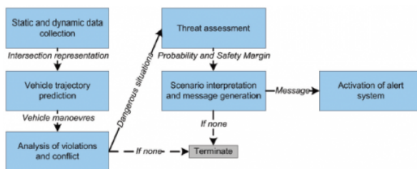
Obrázek 4 - Schematický popis fungování systému IRIS (obr. 5 normy)
