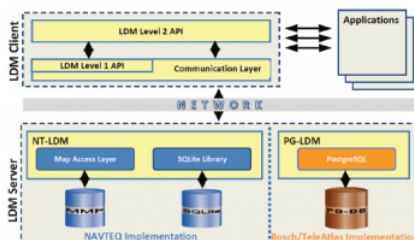
Obrázek 5 - Architektura systému LDM (obr. 9 normy)
