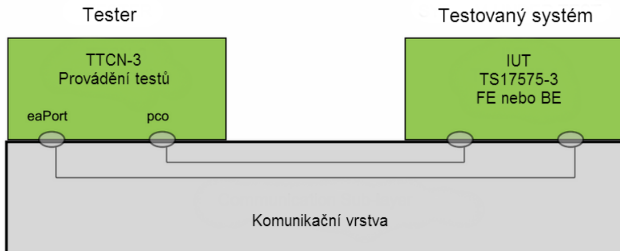
Obrázek 1 - Architektura testovacího systému (obrázek 1 normy)
