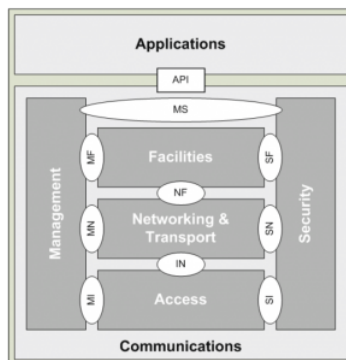
Obrázek 2 normy - Referenční architektura ITS stanice
