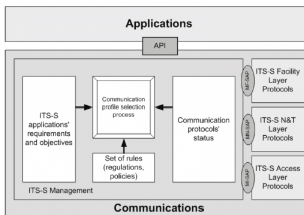
Obrázek 1 normy - Architektura ITS stanice
