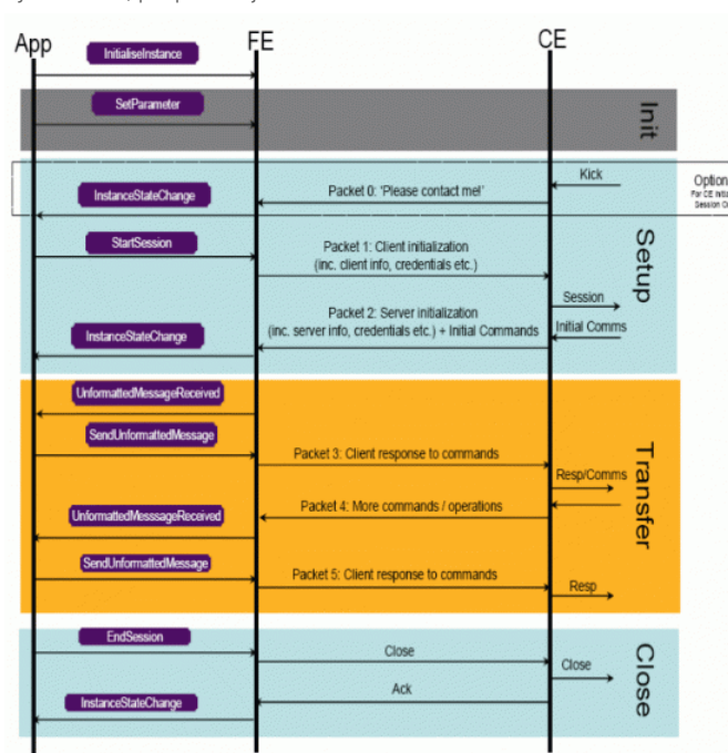
Obrázek 6 - Příklad toku zprávy (relace zahájena od CE)
