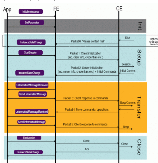
Obrázek 6 - Příklad toku zprávy (relace zahájená od CE)
