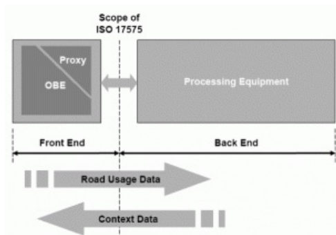
Obrázek 2 – Předpokládaná technická architektura a rozhraní
