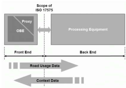
Obrázek 2 - Předpokládaná technická architektura a rozhraní
