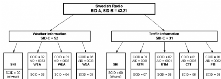
Obrázek 4 - Příklad alokace služeb v národním radiovém přenosovém médiu
