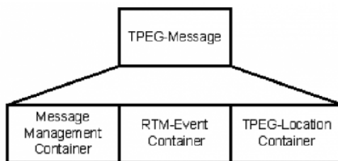
Obrázek 7 – Struktura zásobníků TPEG-RTM
