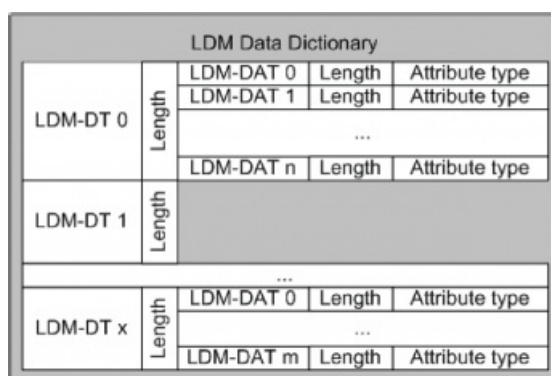
Obrázek č.3 – Koncept LDM datového slovníku
