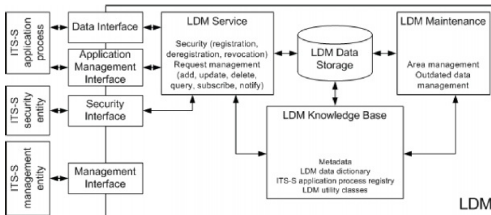
Obrázek č. 2 – Struktura LDM
