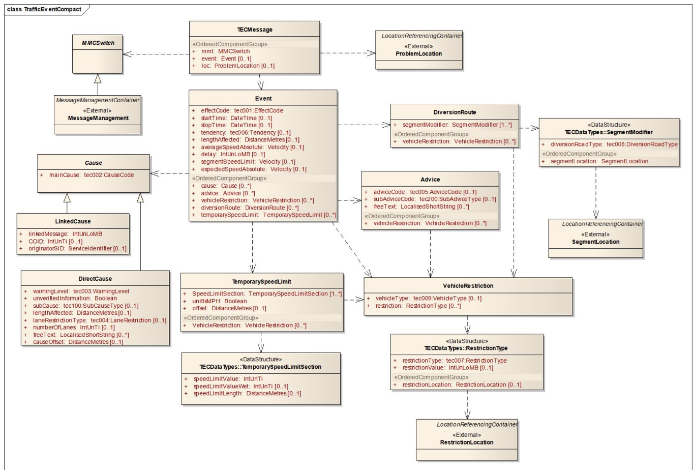
Obrázek 1 - UML model tříd aplikace TEC (obr. 4 normy)
