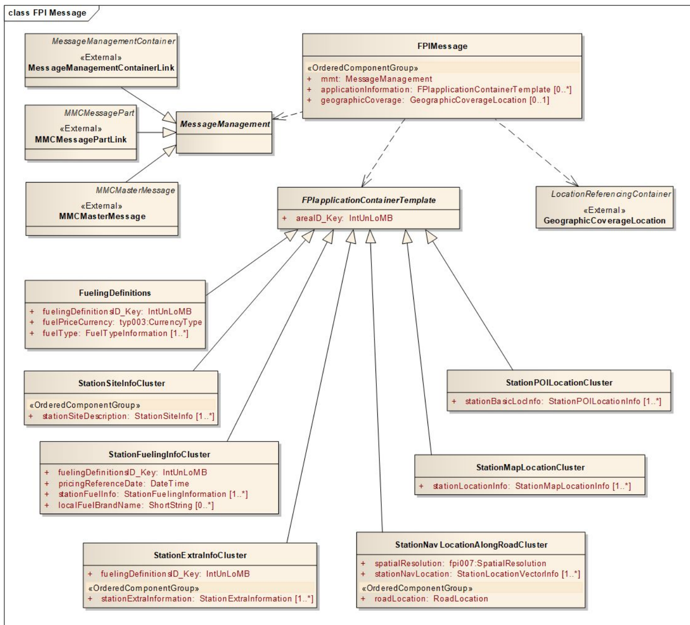
Obrázek 1 – UML model tříd aplikace FPI (obr. 2 normy)
