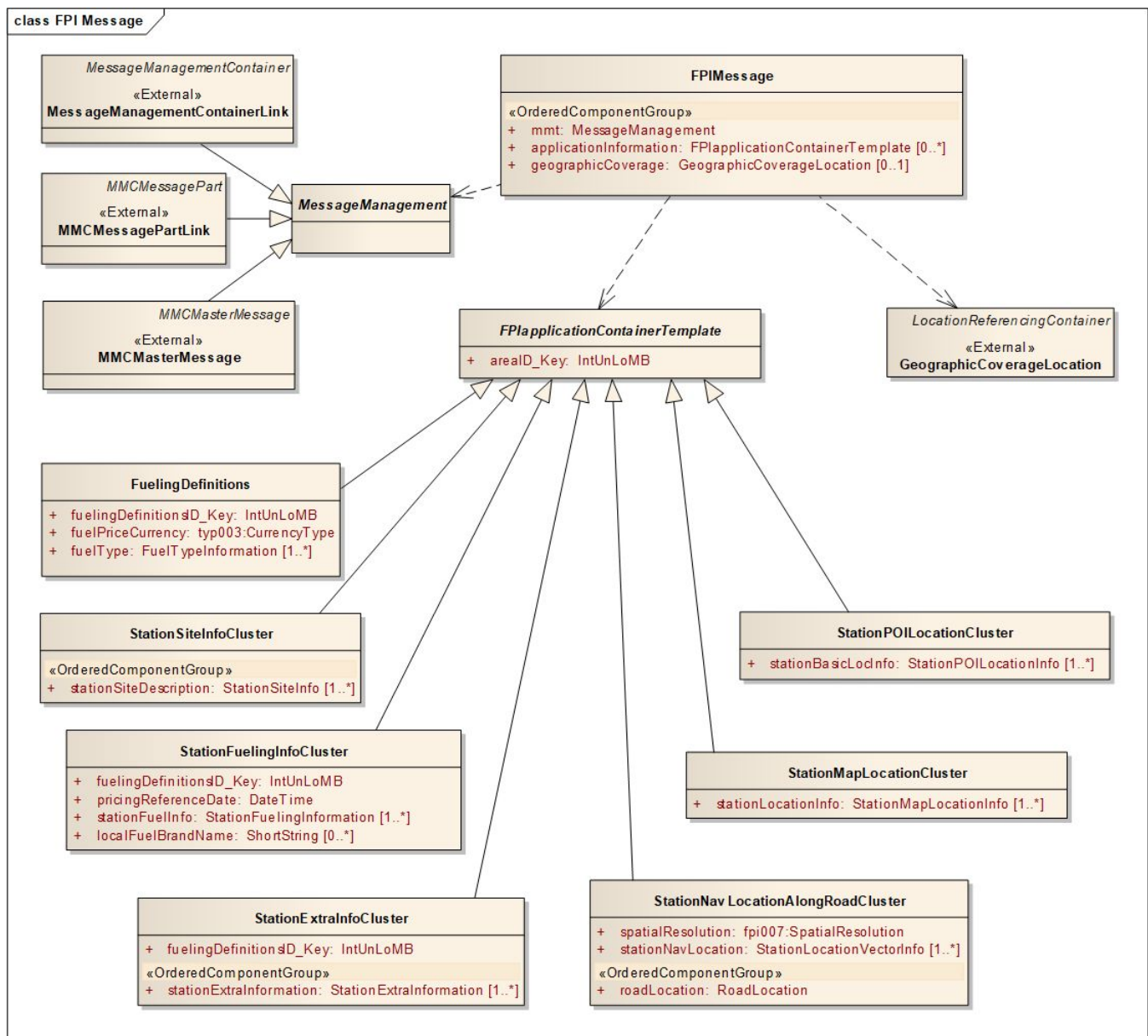
Obrázek 1 - UML model tříd aplikace FPI (obr. 2 normy)
