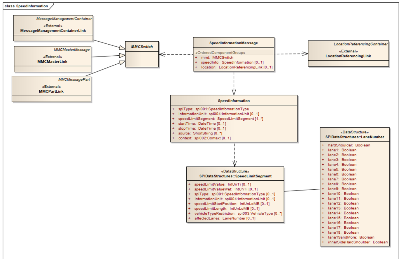
Obrázek 1 - UML model tříd aplikace SPI (obrázek 2 normy)
