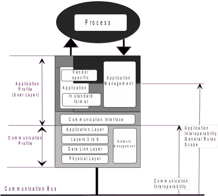
Obrázek A.1 – Model interoperabilního zařízení
