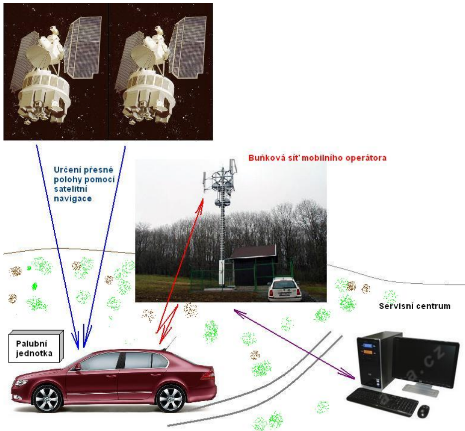
Obrázek A-1 - Přehledné schéma systému
