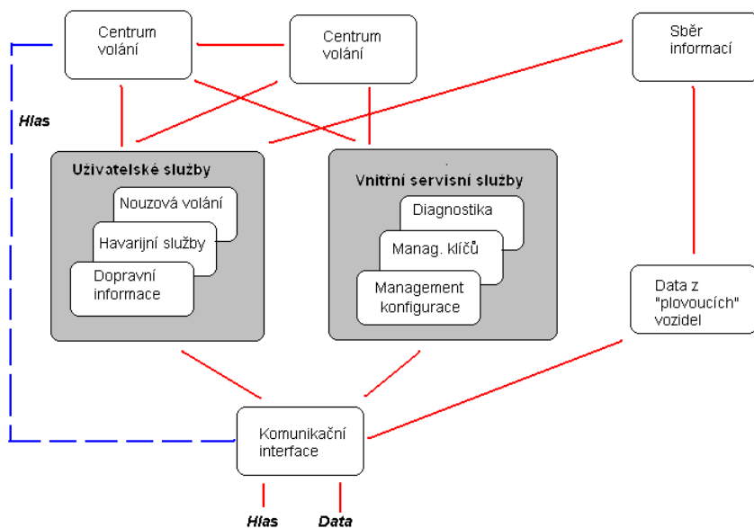
Obrázek A-8 - Logická architektura servisního centra
