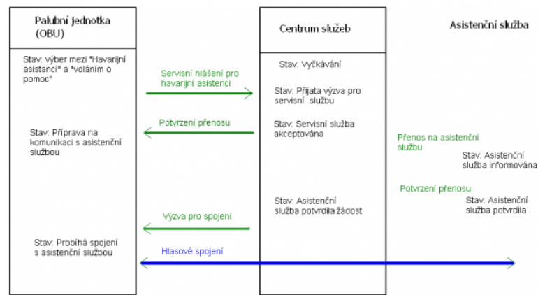
Obrázek 1 – Vývojový diagram komunikace při závadě na vozidle
