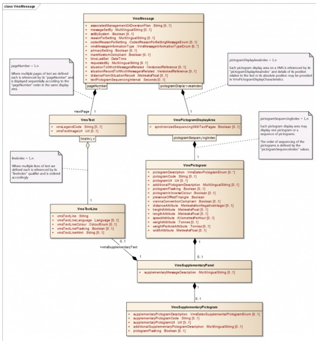
Obrázek 1 – Model tříd balíčku „VmsMessage“ (obrázek 4 normy)
