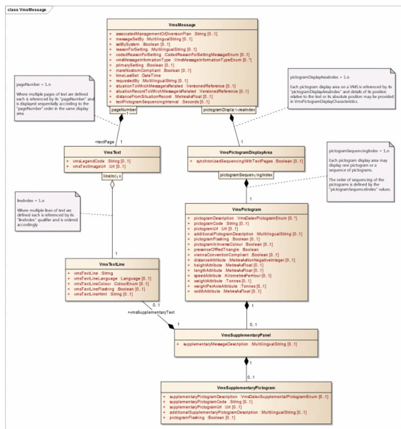
Obrázek 1 - Model tříd balíčku „VmsMessage“ (obrázek 4 normy)
