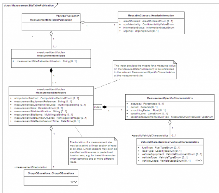
Obrázek 1 - Model tříd balíčku „MeasurementSiteTablePublication“ (obrázek 1 normy)
