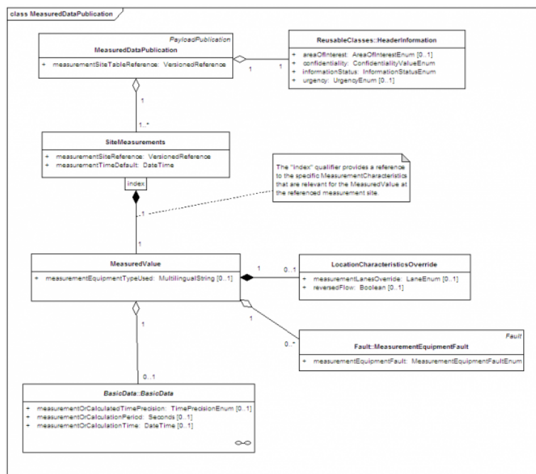
Obrázek 2 – Model tříd balíčku „MeasuredDataPublication“ (obrázek 2 normy)
