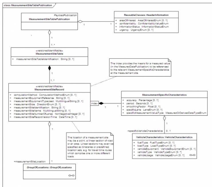
Obrázek 1 - Model tříd balíčku „MeasurementTypeSiteTablePublication” (obrázek 1 normy)
