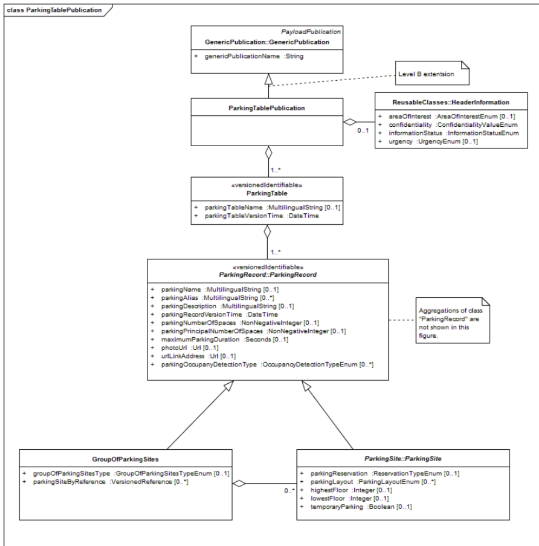
Obr. 1 - Model tříd balíčku "ParkingTablePublication" (obr. 2 normy)
