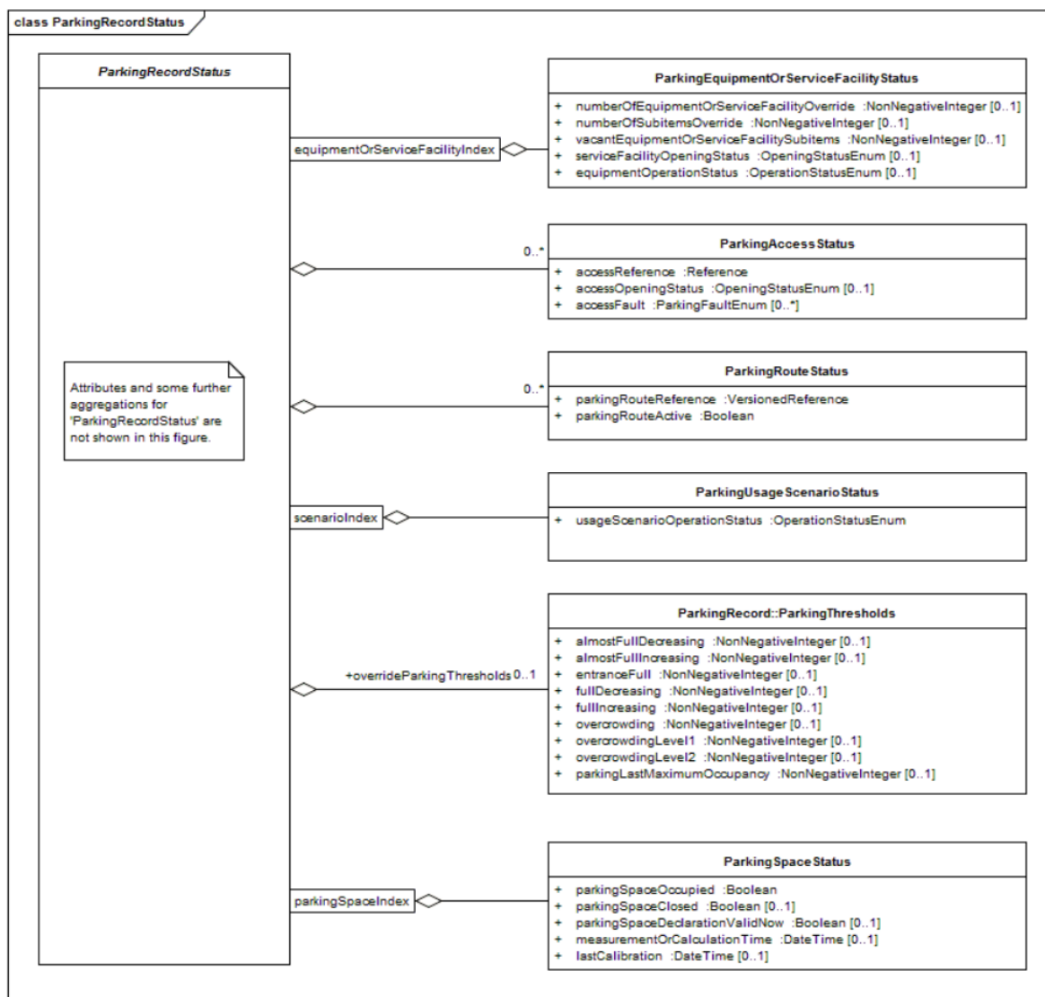
Obrázek 2 - Model tříd balíčku "ParkingRecordStatus" (obr. 21 normy)
