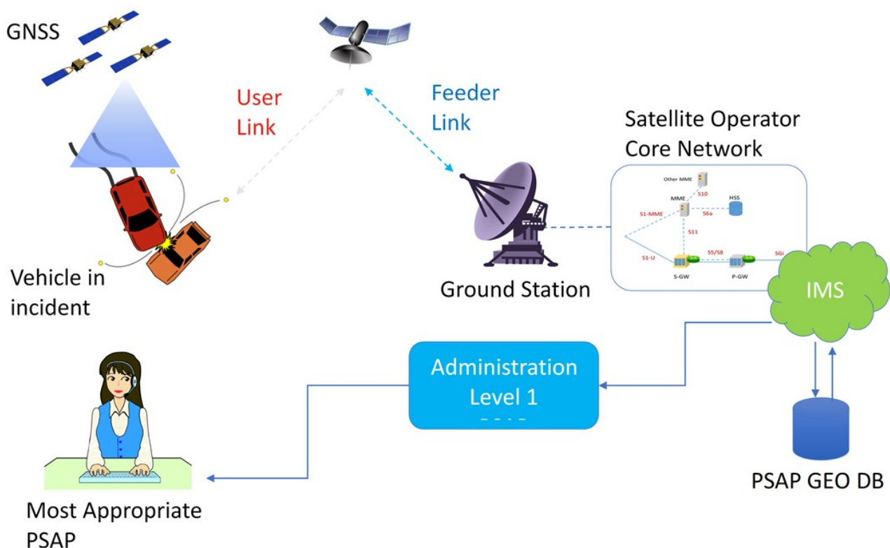
Obrázek 1 - Satelitní síť podporující IP a IMS v hlavní (core) síti
