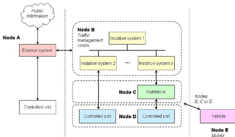
Obrázek 4 – UTM model uzlových bodů (obr. C.2 normy)
