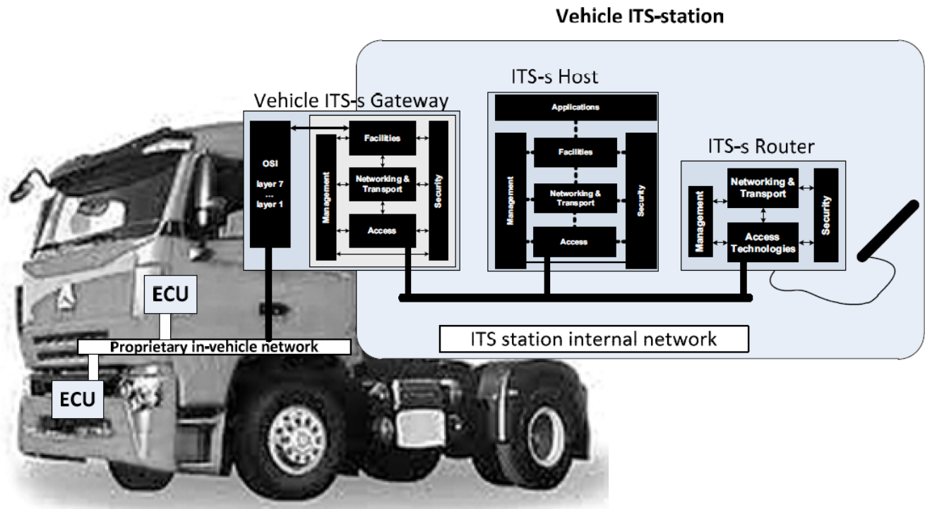
Obrázek 2: Subsystem ITS ve vozidle (obrázek 3 normy; zdroj: ISO 21217 )
