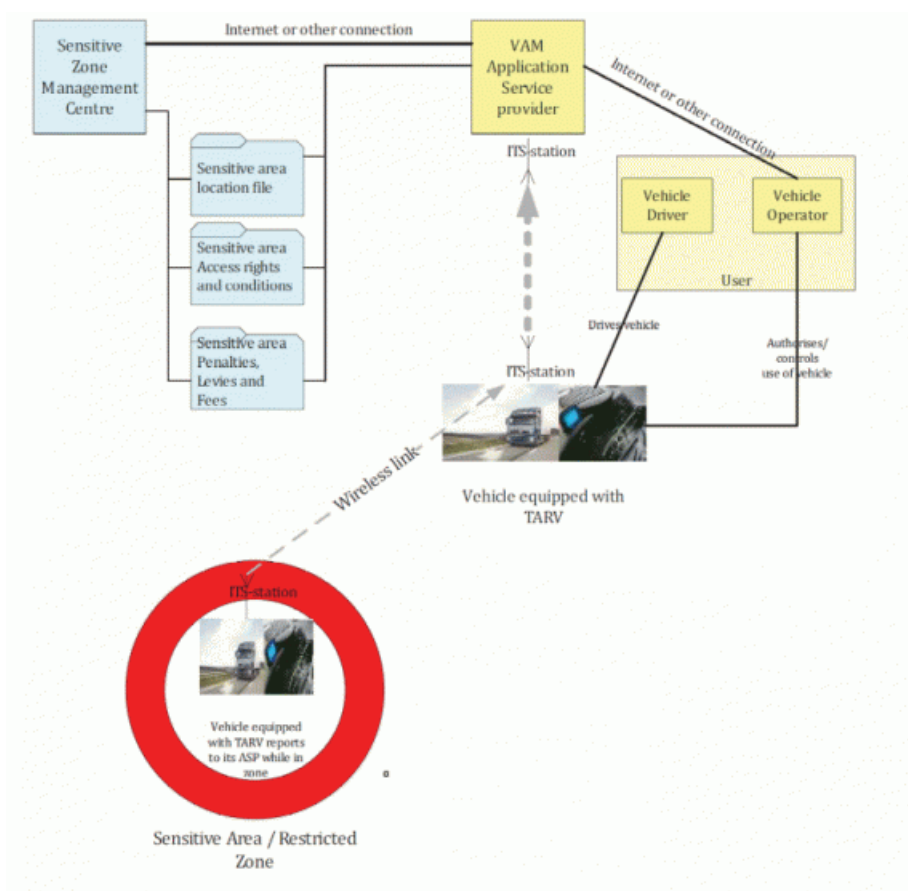
Obrázek 1 – Přehled monitorování vjezdu vozidla (Obrázek 2 normy)
