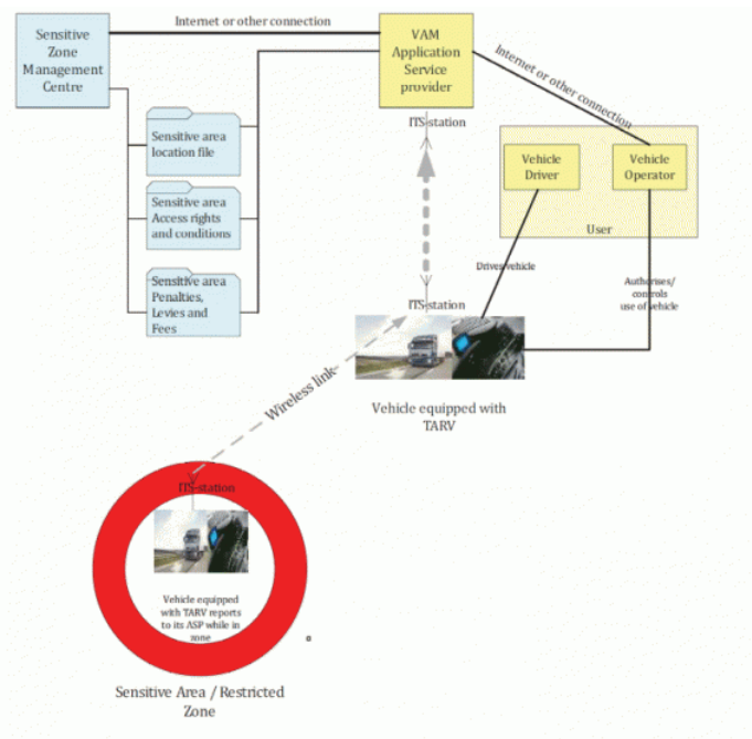
Obrázek 1 – Přehled monitorování vjezdu vozidla (Obrázek 2 normy)
