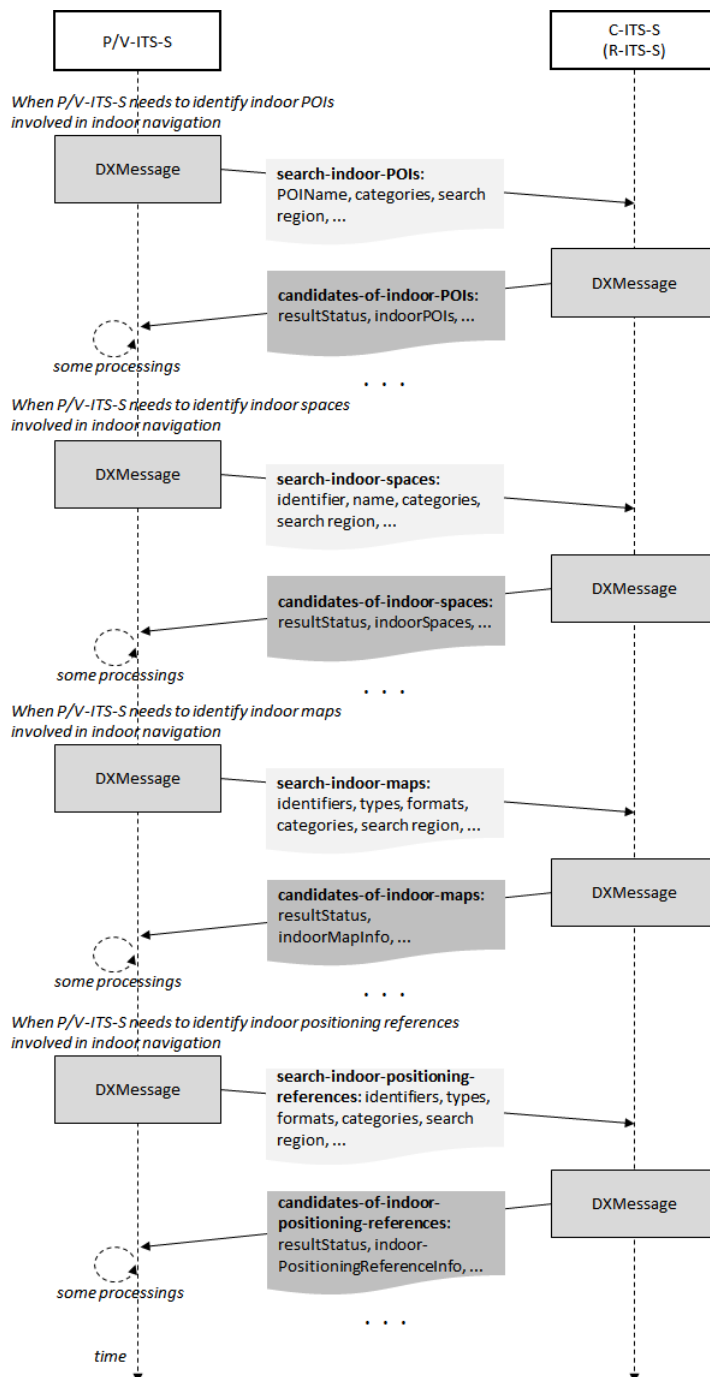
Obrázek 2: Vývojový diagram zpráv (obrázek 2 normy)
