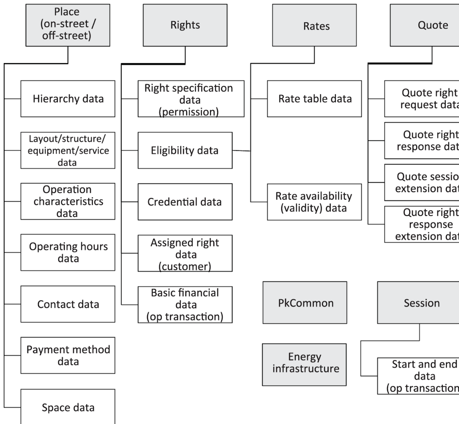
Obrázek 1 - Datové domény parkování (obrázek 1 normy)
