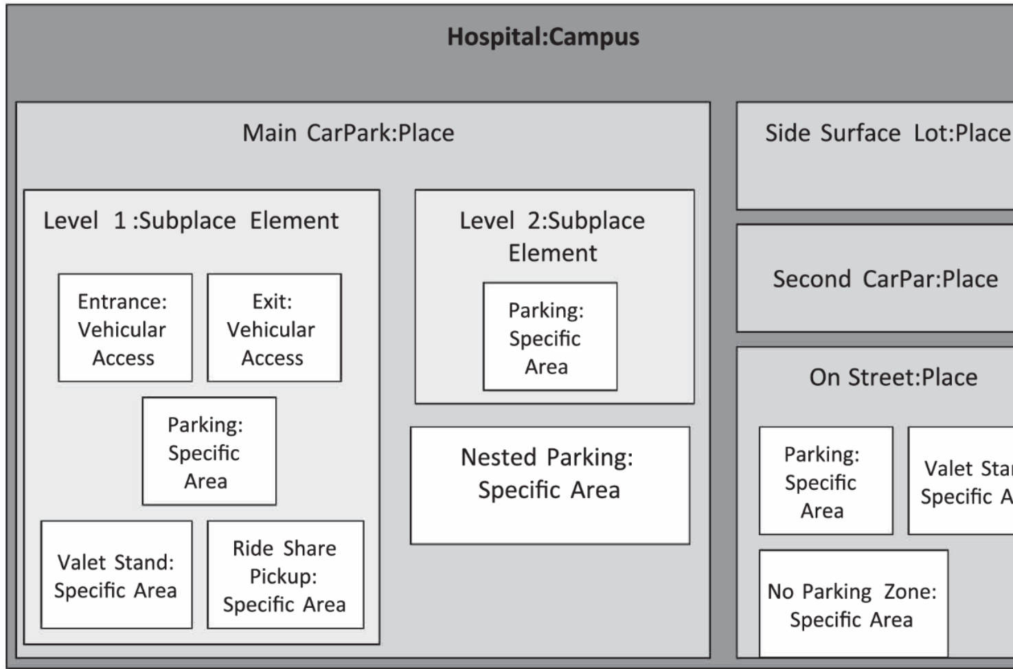
Obrázek 2 – Datové domény parkování (obrázek 3 normy)
