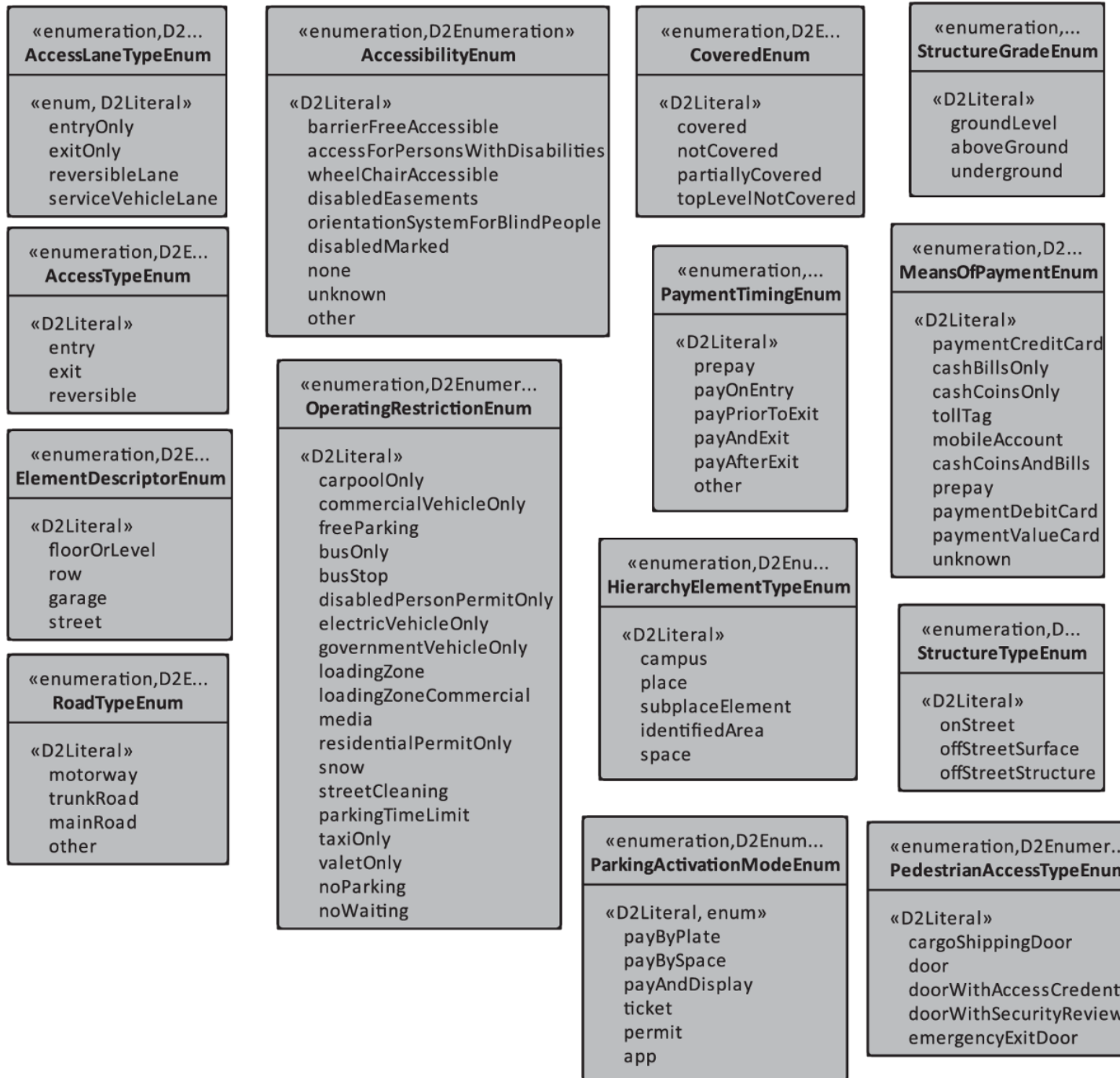
Obrázek 4 – Číselníky v doméně Place (obrázek 17 normy)
