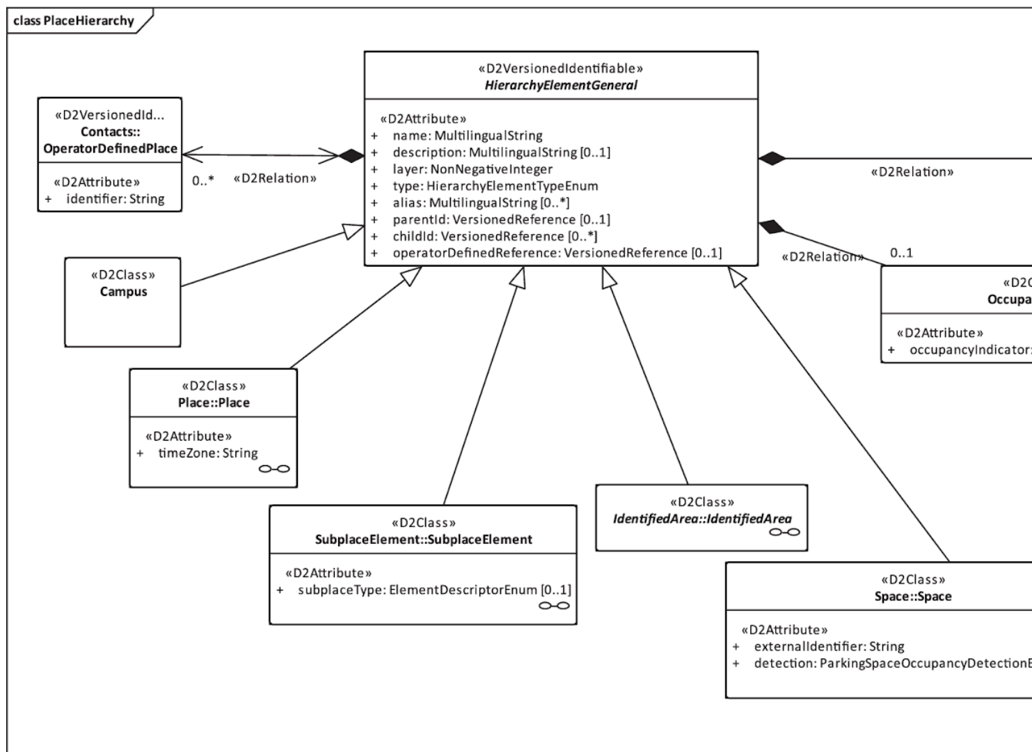
Obrázek 3 - Hierarchie domény Place (obrázek 4 normy)
