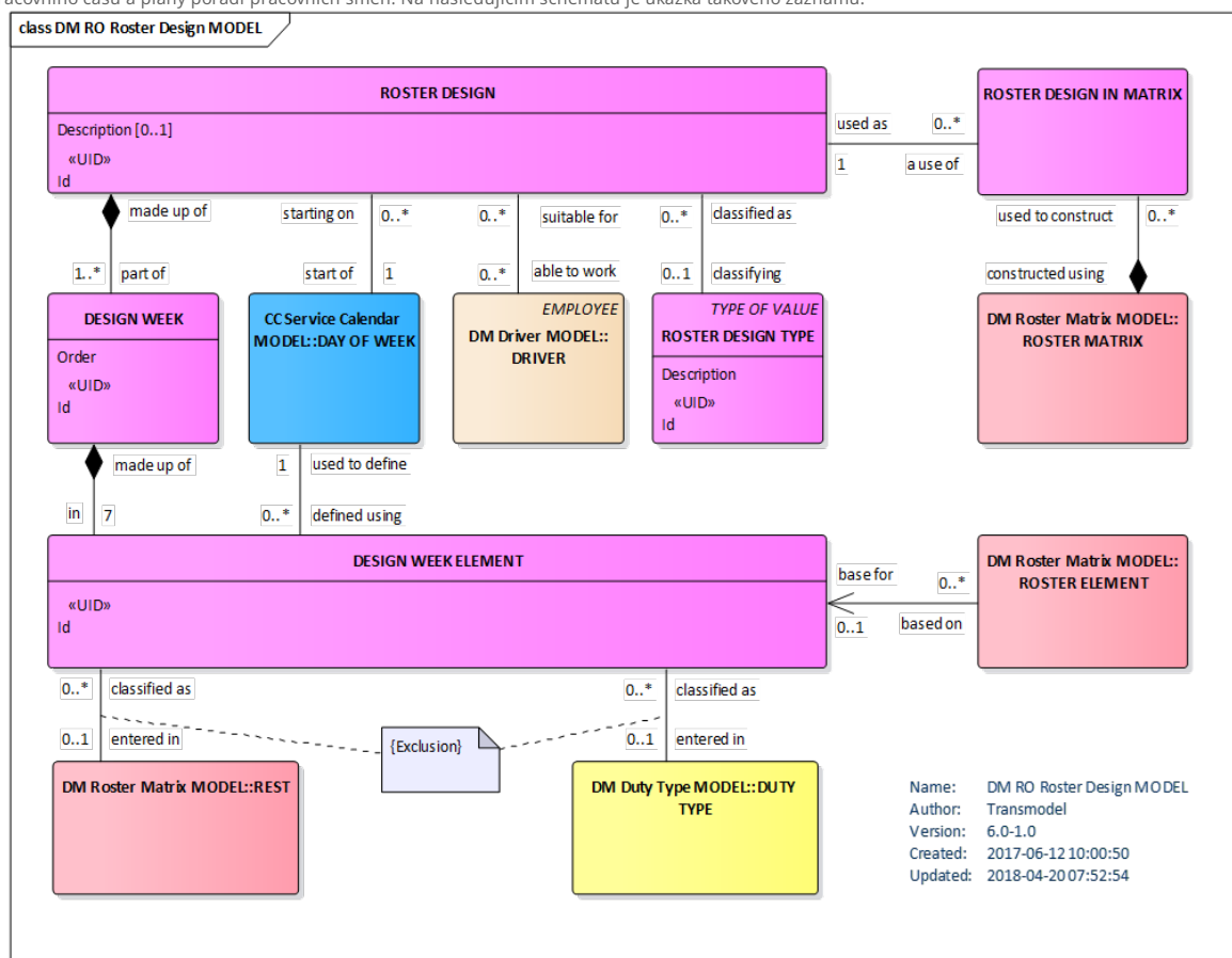
Obrázek 2 – UML model - Matice přiřazení povinností (obr.18 normy)
