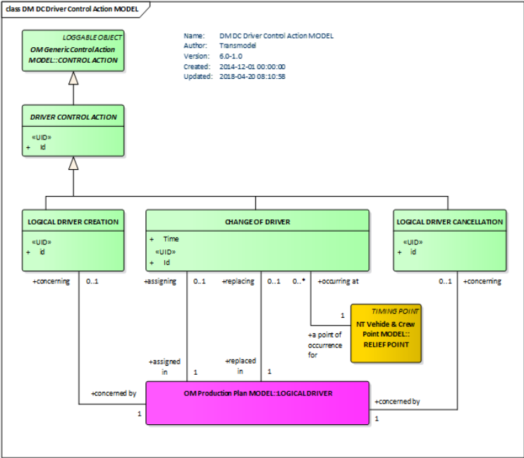
Obrázek 3 –UML model - Denní operativa v rozvrhu řidičů (obr.21 normy)
