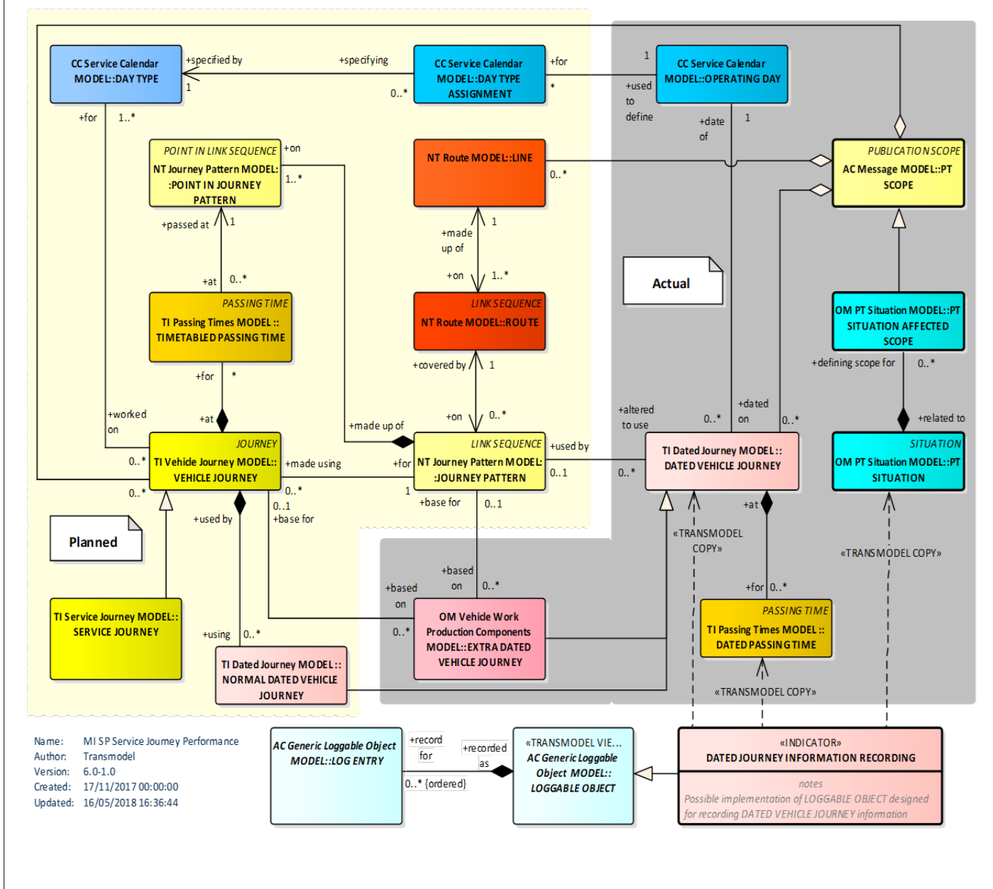
Obrázek 2 – Příklad UML – výkonnost služební jízdy (obr. 9 normy)
