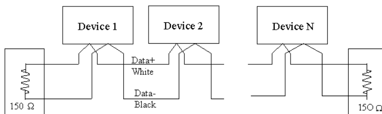
Obrázek 1 - Zapojení mezi zařízeními
