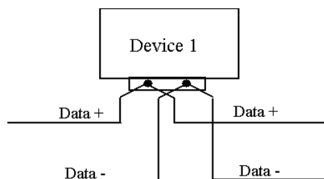
Obrázek 2 - Zapojení pro možnost vyjmutí zařízení , bez narušení funkce sběrnice
