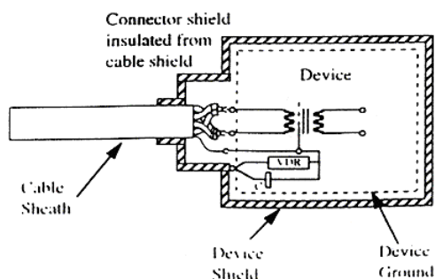
Obrázek 6 - Spojení stínění s kostrou v rámci zařízení
