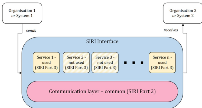
Obrázek 1 - Struktura SIRI: soubor volitelných specifikací rozhraní služeb využívajících společný jazyk (obr. 1 normy)
