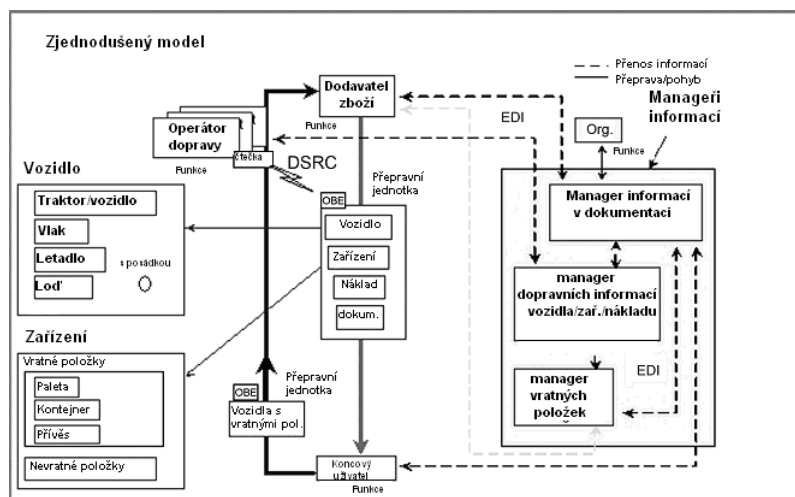
Obrázek A.4 – Koncepční model systému AVI/AEI ukazující jeho třídy a klíčové definice
