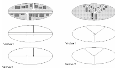
Obrázek 4 – Reprezentace vícepruhové Tří-valenční křižení se třemi spojeními komunikace na Vrstvě 2 a jednou křižovatkou
