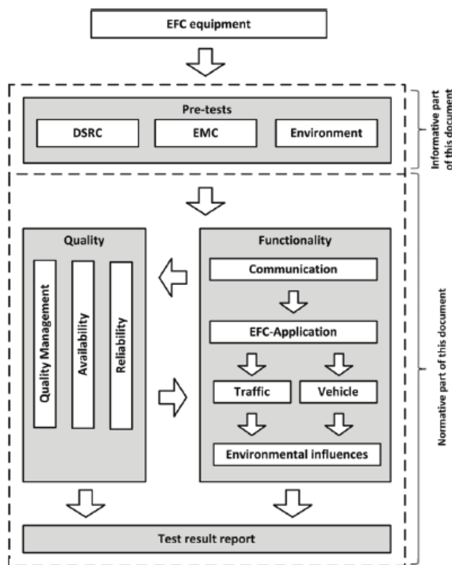
Obrázek 1 – Závislosti zkoušek (obr. 3 normy)
