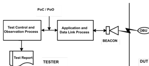
Obrázek 2 - Systém pro zkoušení shody (obr. 5 normy)
