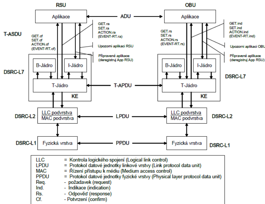
Obrázek 3 - Kontext a struktura jádra aplikační vrstvy
