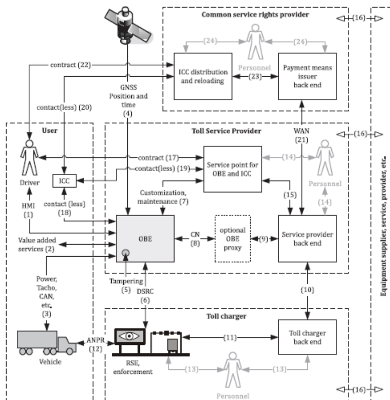
Obrázek 1 – Uvažovaný model pro analýzu hrozeb (obr. D.1 normy)
