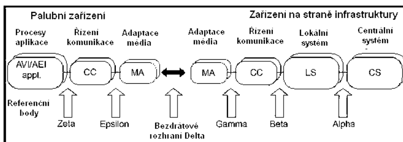
Obrázek 2 - Jednoduché konceptní schéma referenčního modelu architektury systému AVI/AEI (obr. 5 popisovaného dokumentu)
