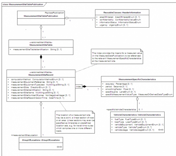
Obrázek 1 - Model tříd balíčku „MeasurementTypeSiteTablePublication” (obrázek 1 normy)
