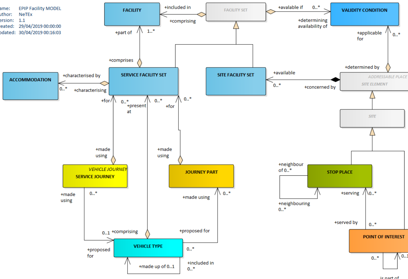
Obrázek 1 - Model vybavení zastávky (obr. 6 normy)
