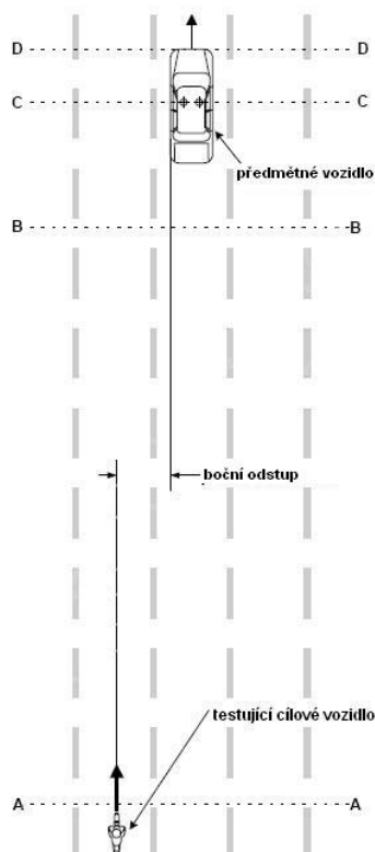
Obrázek 9 - Test - cílové vozidlo předjíždí předmětné vozidlo
