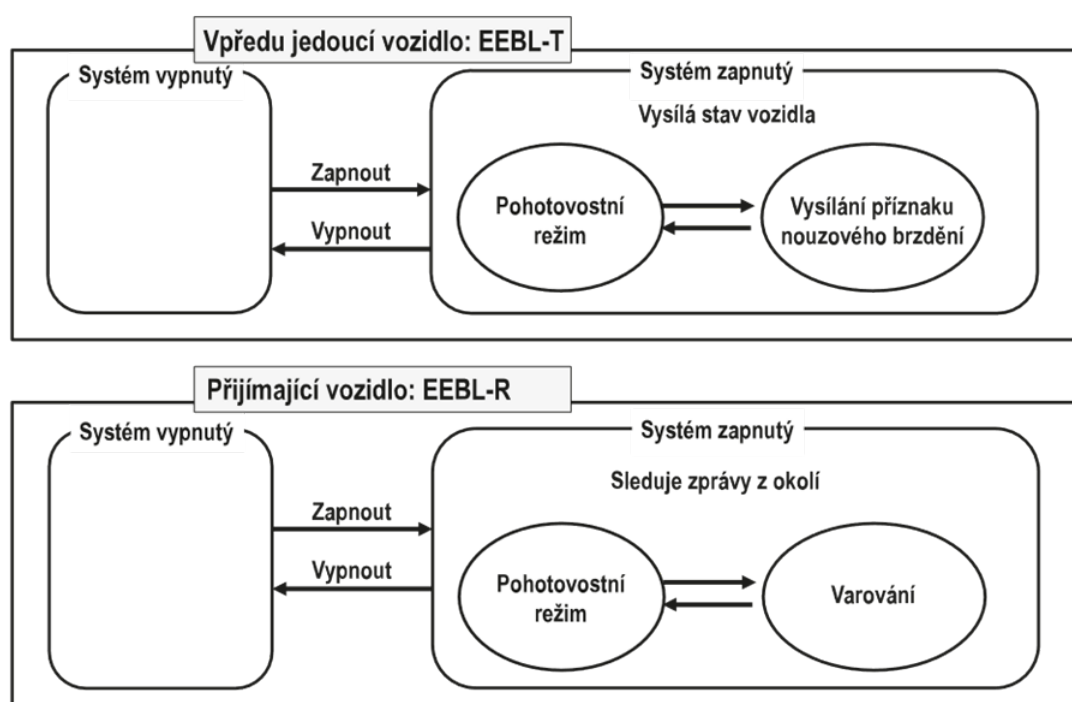
Obrázek 1 (Obrázek 1 normy) - Systém EEBL - diagram stavů a přechodů
