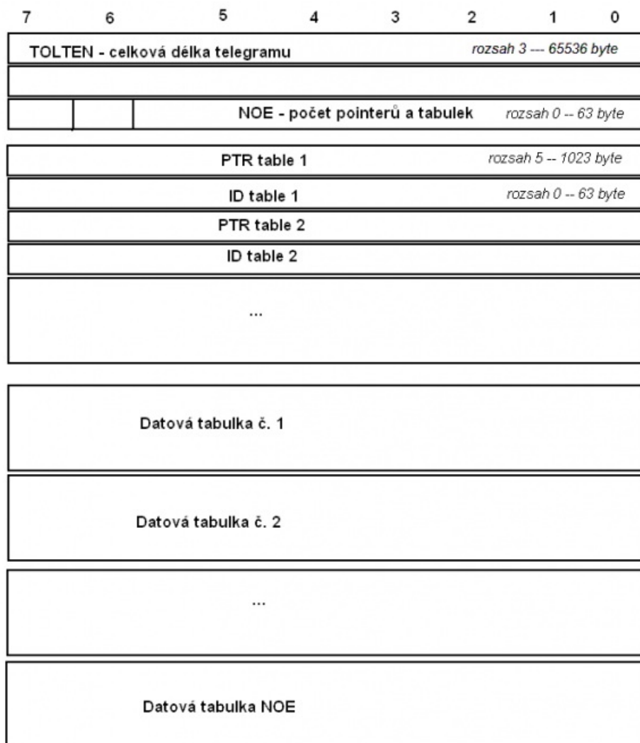
Obrázek 1 – Struktura telegramu
