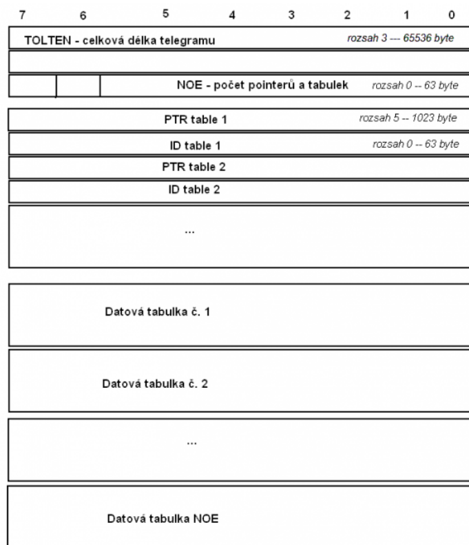
Obrázek 1 - Struktura telegramu
